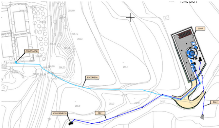
Captació, connexió a serveis i ubicació depuradora.
